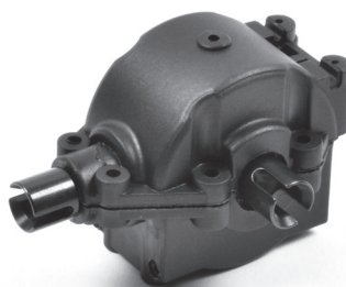
T4905/6 Vorderer Antriebssatz
