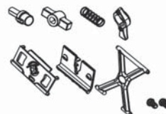
T4972/72 Partie arrière arceau
