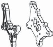
T4972/76 Supports amortisseurs AV/AR
