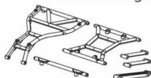
T4972/68 Mittelteil Überrollbügel
