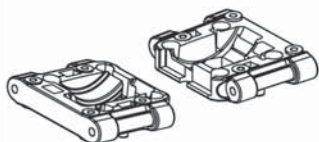
T4971/02 Untere Querlenker- halterungen VO/HI
