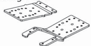
T4972/20 Stahl Chassisverstär- kung VO/HI
