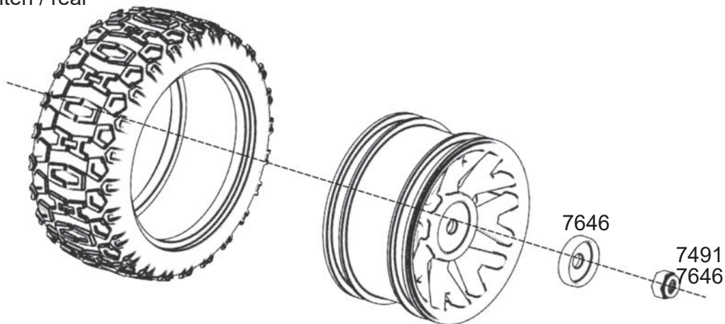
7486 hinten / rear
