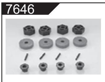
7646 Radmitnehmer, Pins, Muttern, Unterlegscheiben (Kunst- stoff) (je 4x)
