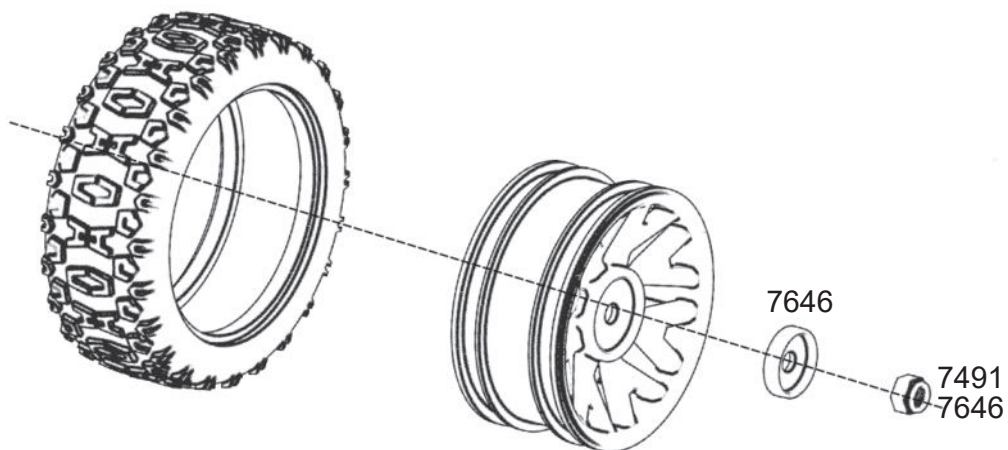
7485 vorne / front
