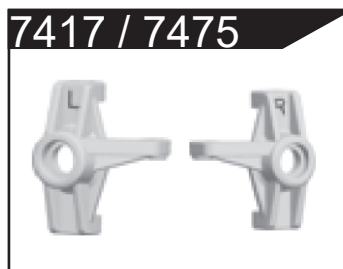
7417 / 7475 Lenkhebel vorne (2) 7417 - Kunststoff 7475 - Metall
